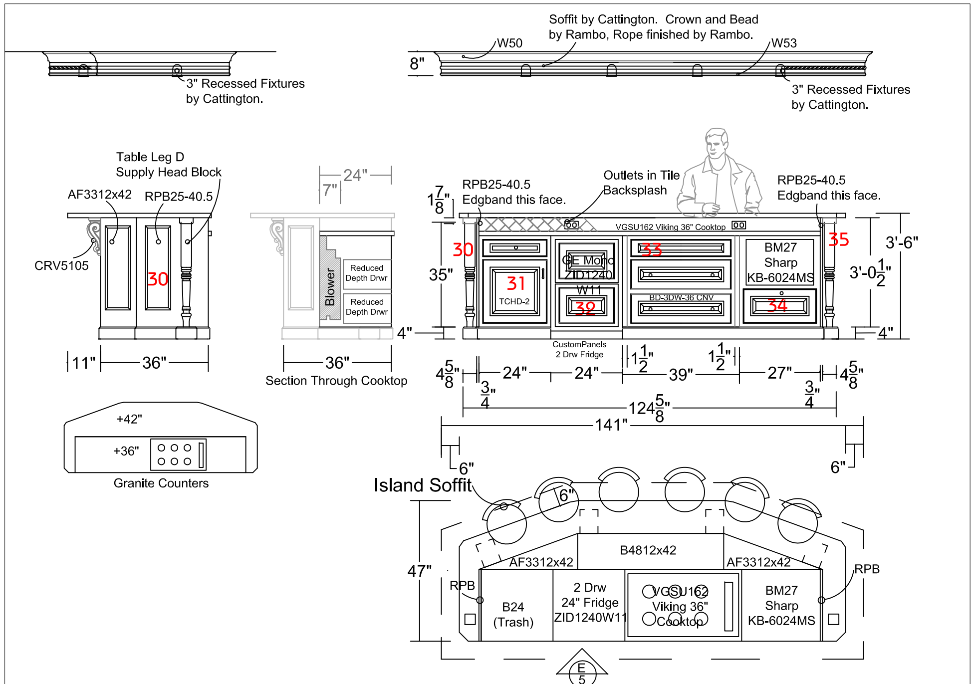
1 Elevation E Scale: 3/8" = 1'-0"
