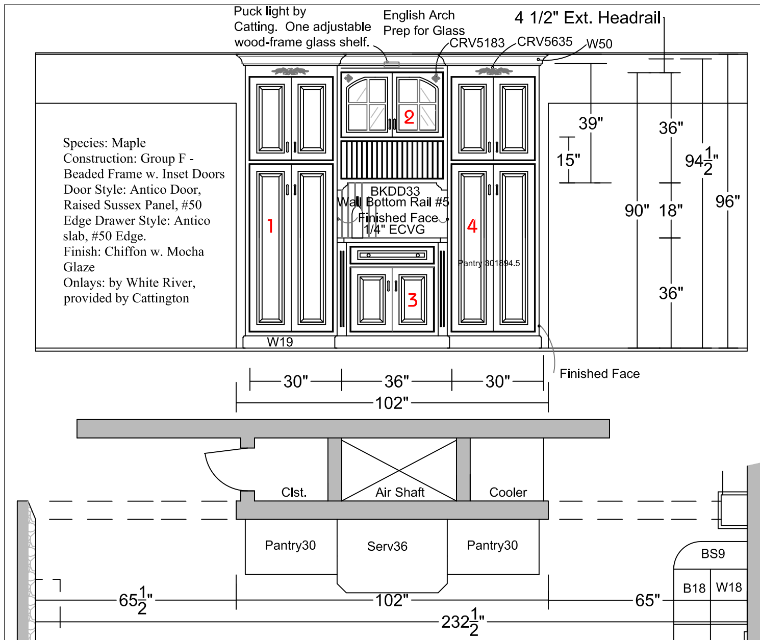
1 Elevation A Scale: 3/8" = 1'- 0"
