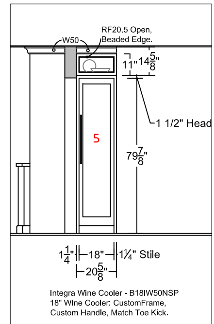
1 Cooler Elevation Scale: 1/4" = 1'- 0"
